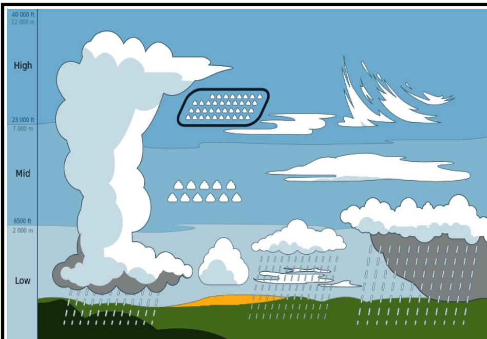
cirrocumulus
