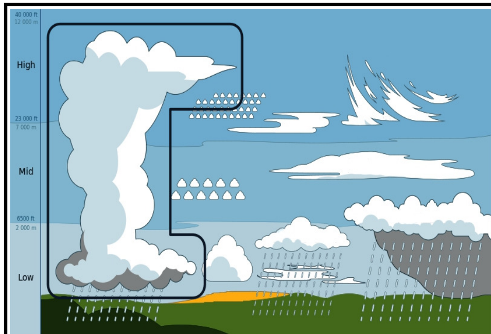
cumulonimbus
