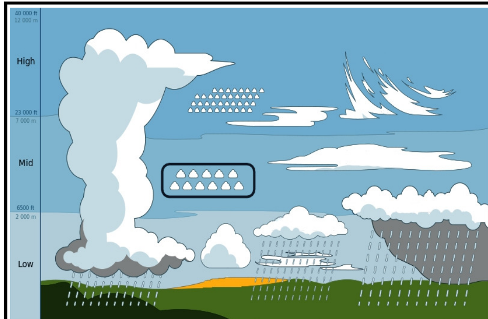
altocumulus
