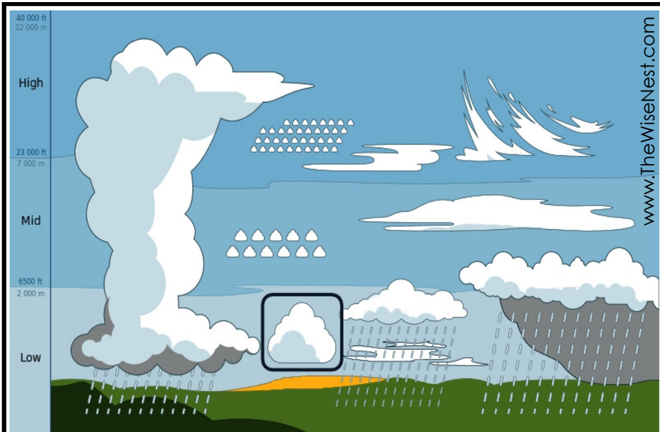
cumulus
