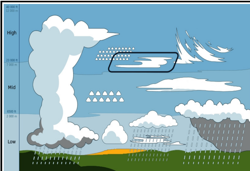
cirrostratus
